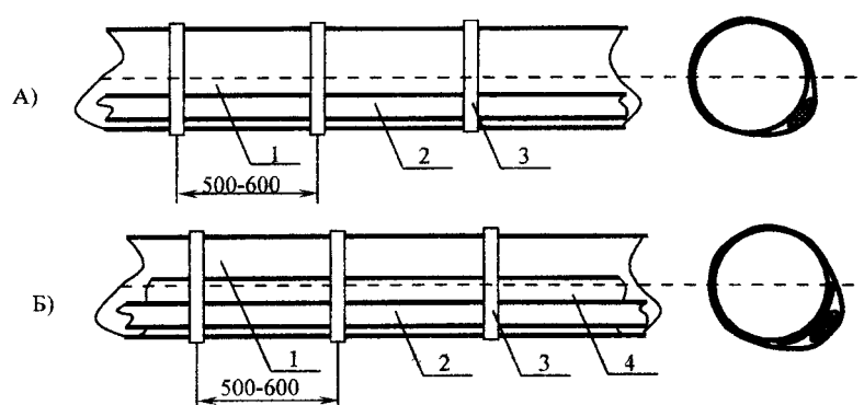
А) прокладка кабеля по металлической трубе; Б) прокладка кабеля по пластмассовой трубе 1 — труба; 2 — нагревательный кабель; 3 — поясик из ленты с липким слоем (2-3 витка); 4 — лента алюминиевая с липким слоем
