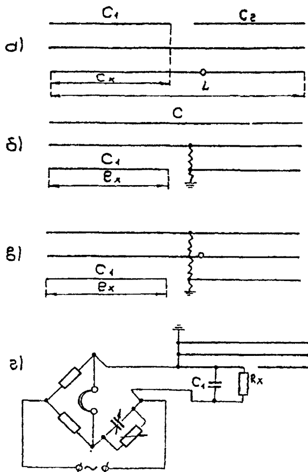
а, б, в) Виды повреждений кабелей; г) Схема для определения емкости Рисунок 11.1
