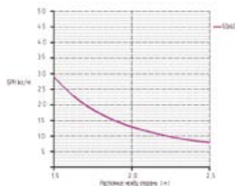
График нагрузки
