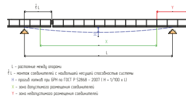
Размещение креплений
