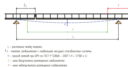
Размещение креплений
