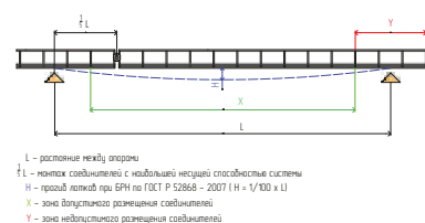
Размещение креплений
